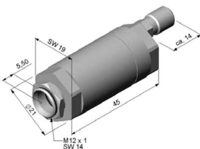
Standard-Freiblasvorsatz, kombinierbar mit Montagewinkel
