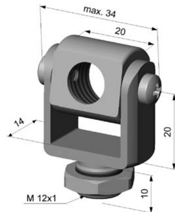
Montagegabel mit M 12x1-Gewinde, justierbar in 2 Achsen
