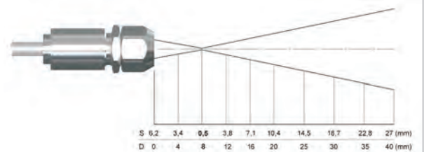
25:1 Optik mit CF-Vorsatzlinse
